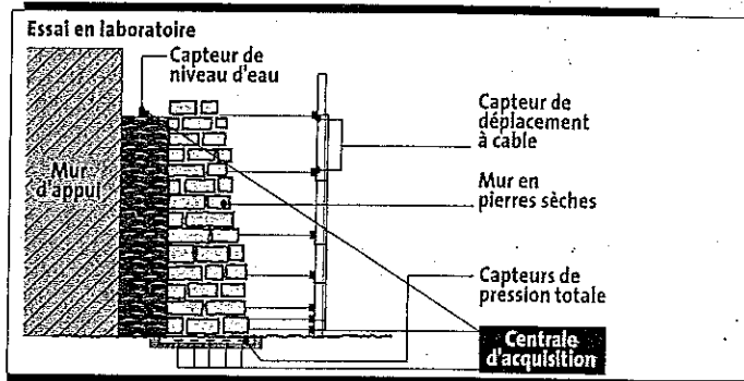
Schéma de principe du chargement par pression d'eau
